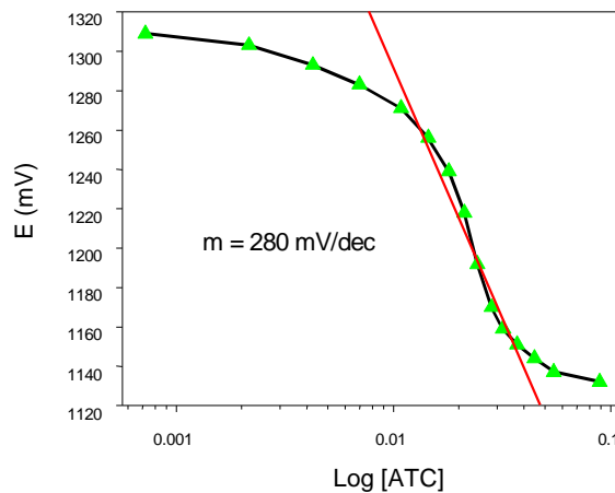
Figura 10. Gráfica de potencial del EnFET respecto de la concentración de acetilcolina.
