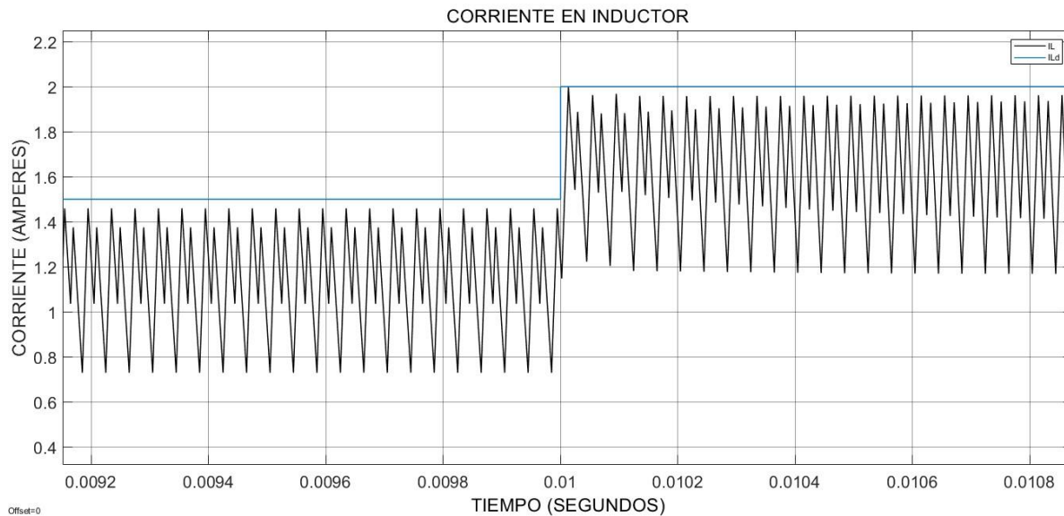
Figura 4. Regulación de la corriente en el inductor.
