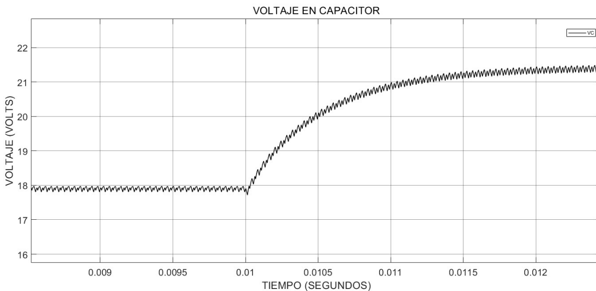
Figura 5. Voltaje del capacitor.
