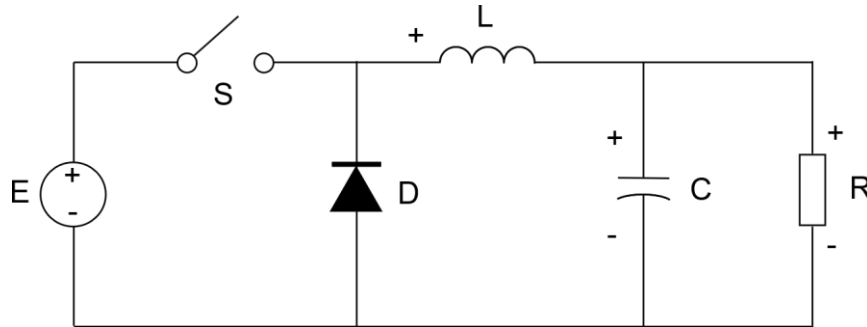
Figura 1. Convertidor reductor ideal.
